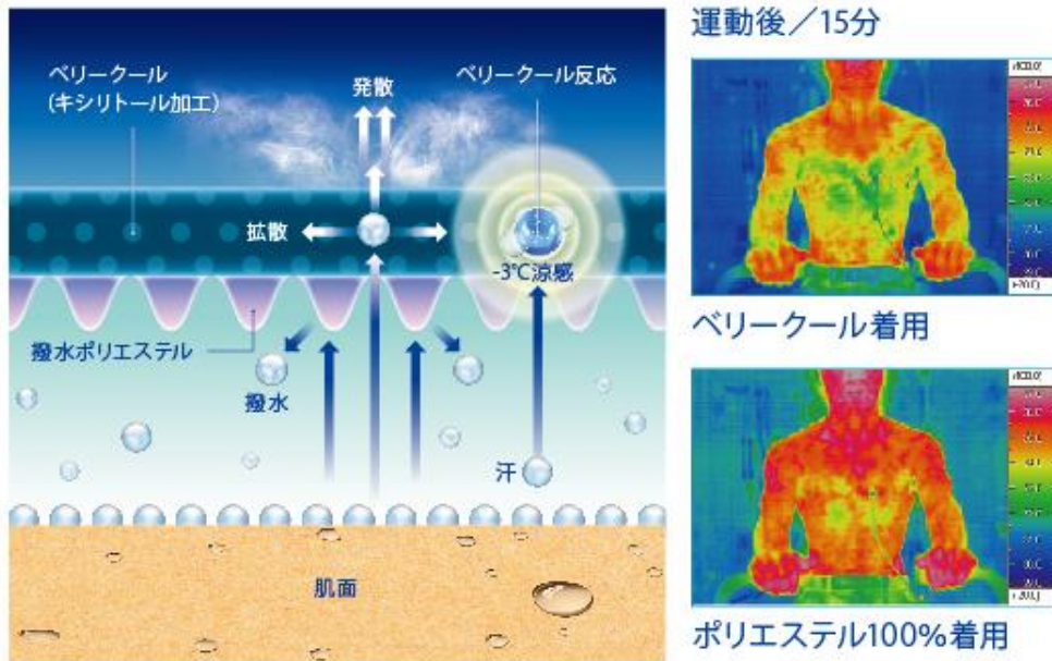
(左)ベリークールドライ機能図解 (右)サーモグラフィーを用いたベリークールの比較実験 ユニチカガーメンテック(株)計測データ
