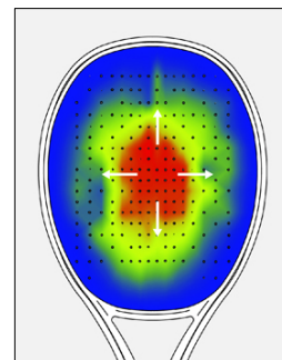
【ストリング振動モード解析図】 赤い部分が最も反発の高いゾーンで、これが縦横に拡大した（ヨネックス調べ）
