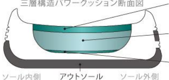
三層構造パワークッション断面図
